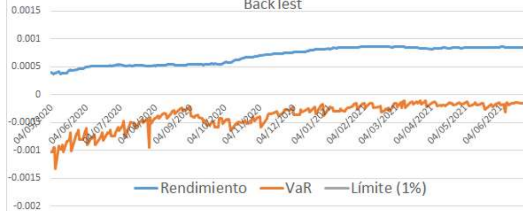
BackTest
