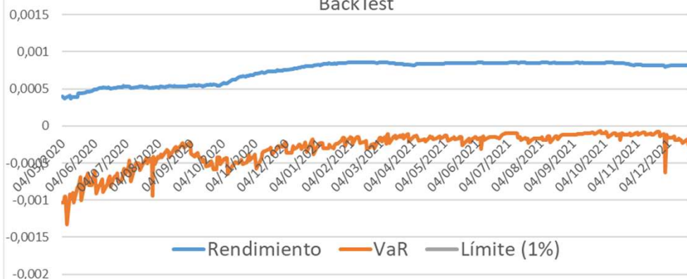
BackTest
