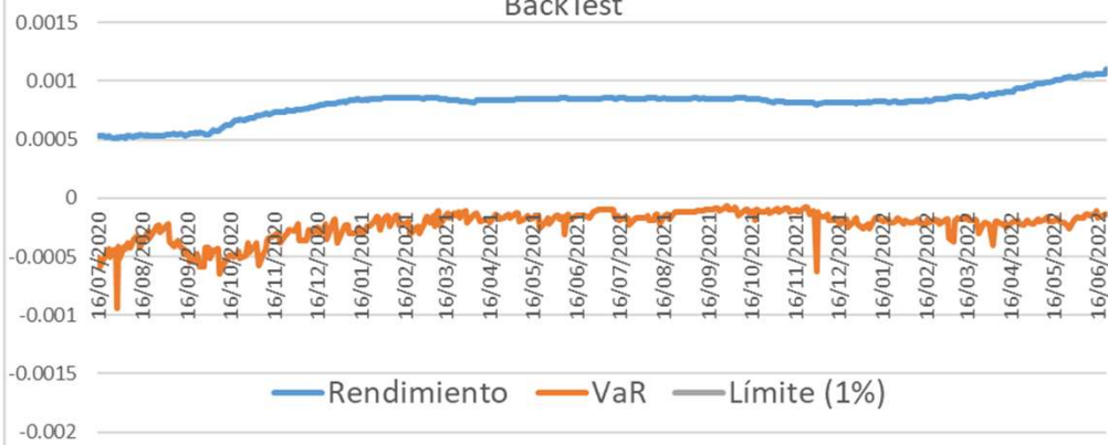
BackTest
